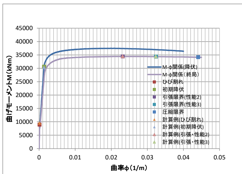
図 20-4 道示 V に基づく M-\phi 関係の計算例（矩形断面・橋軸方向）
