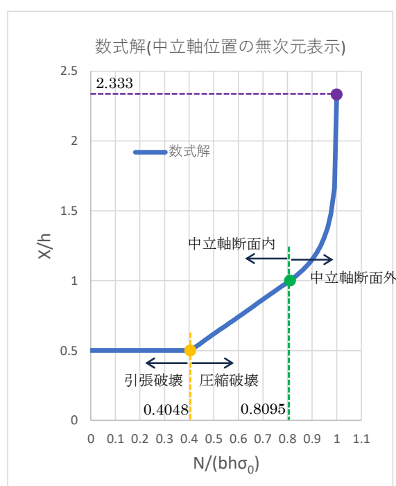
(b) 中立軸位置
