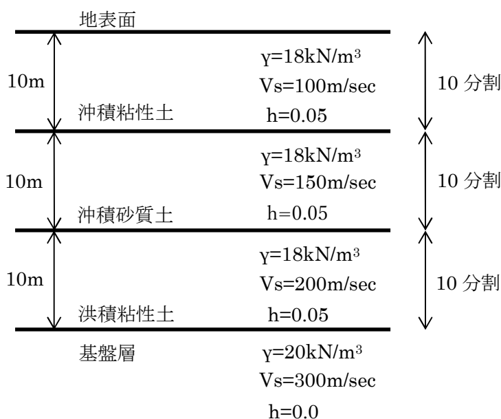
図 15-1 計算例の地層構成
