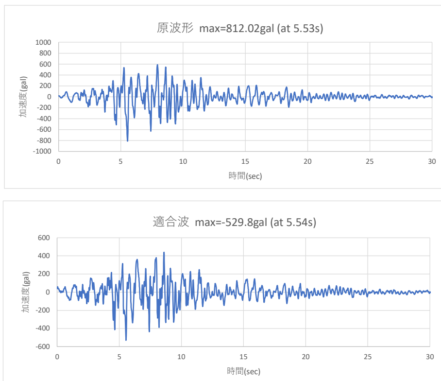
図 26-2 原波形と適合波形
