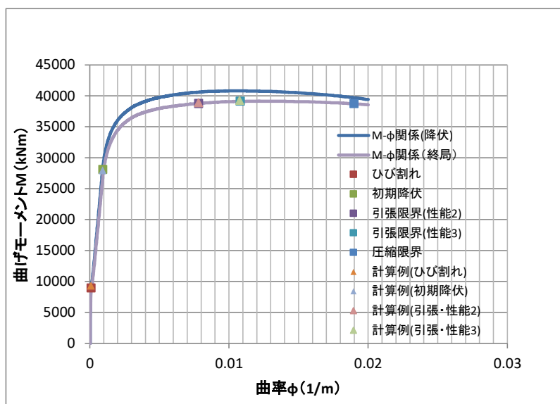
図 20-3 道示 V に基づく M-\phi 関係の計算例（円形断面）
