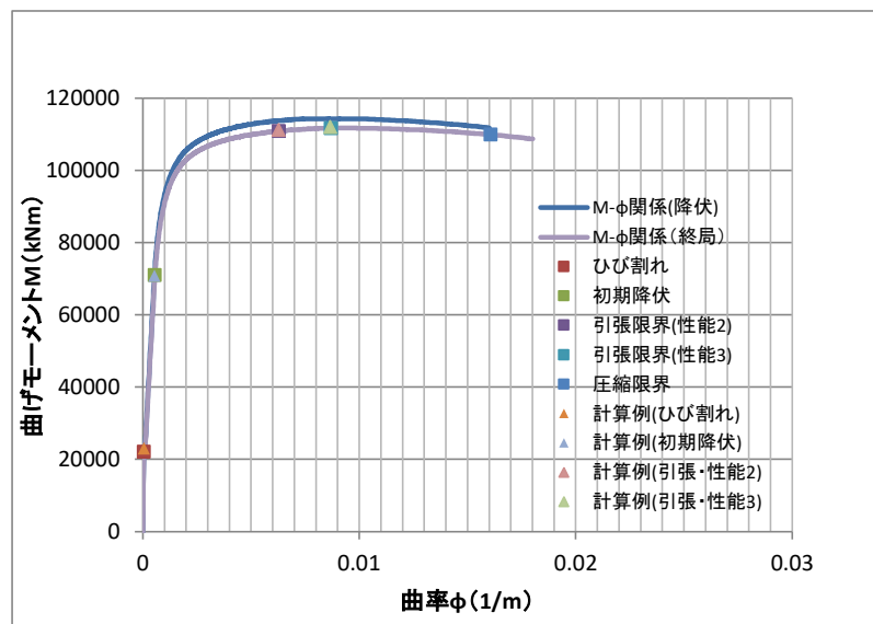
図 20-7 道示Vに基づく M-\phi 関係の計算例（小判形断面・長辺方向）
