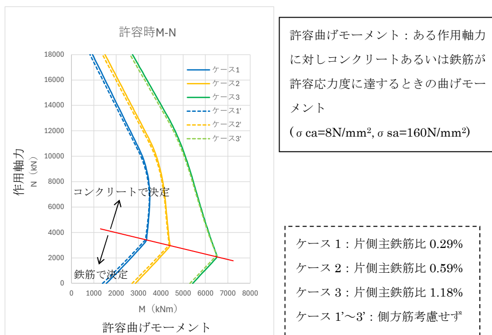
図 2-1 許容時 M-N 関係
