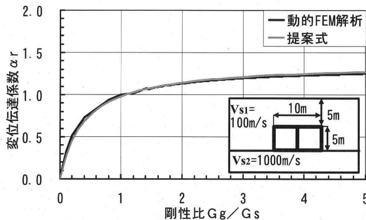
(b)変位伝達係数 \alpha_r と剛性比 G_g/G_s の関係
