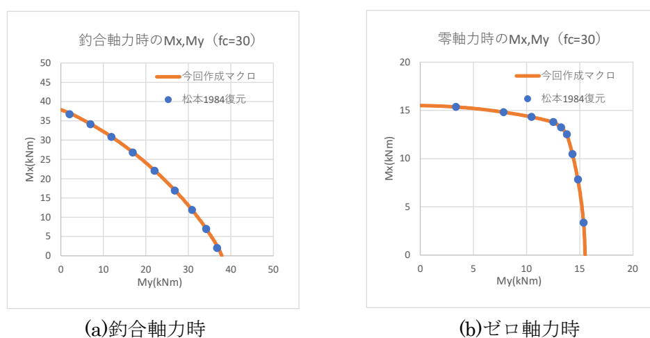
図 13-1 M_x - M_y 関係
