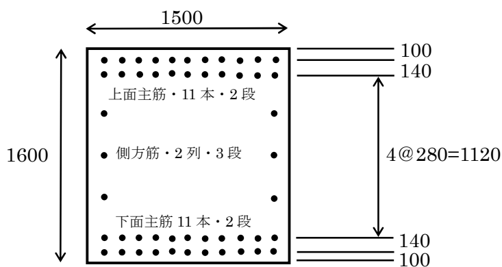
図 2-2 鉄筋配置
