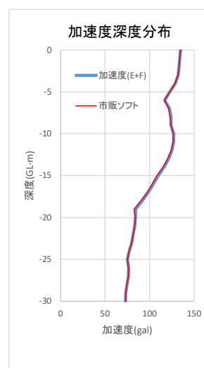
(b) 加速度深度分布
