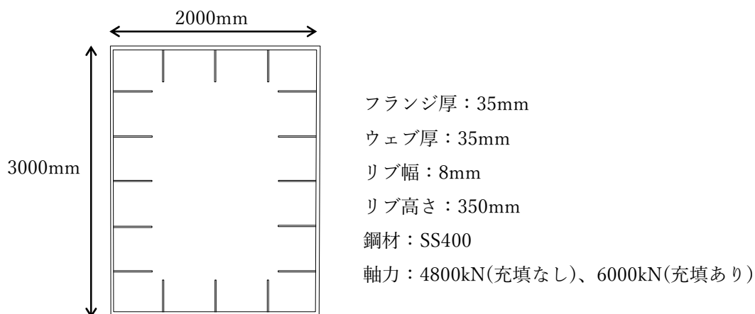
図 21-1 計算対象とした矩形鋼断面
