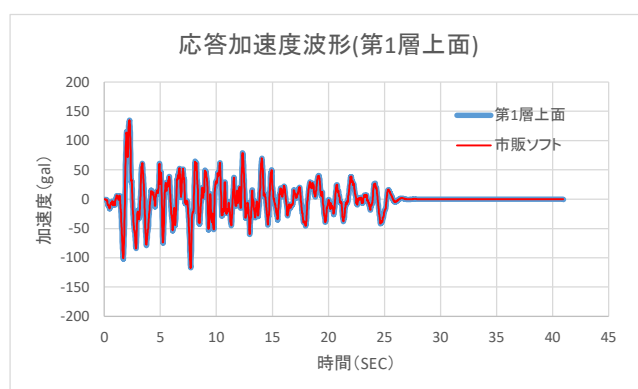
(a) 応答加速度波形
