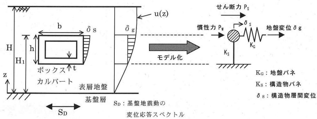
(a)地震時変形量を推定するための解析モデル
