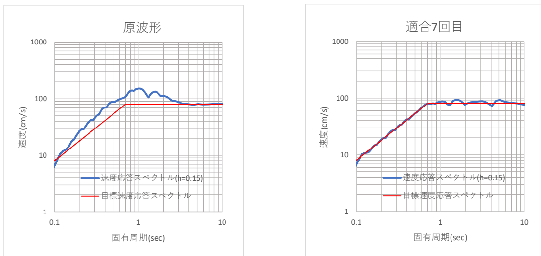
図 26-1 目標応答スペクトルとの適合
