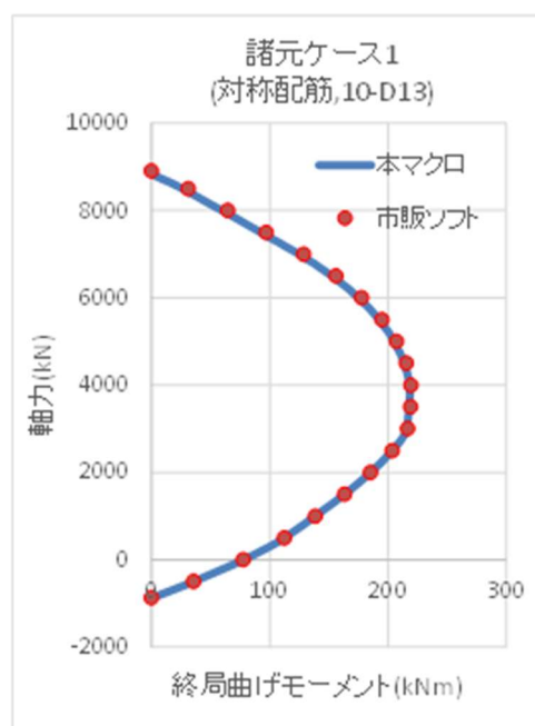
(b) 市販ソフトとの比較
