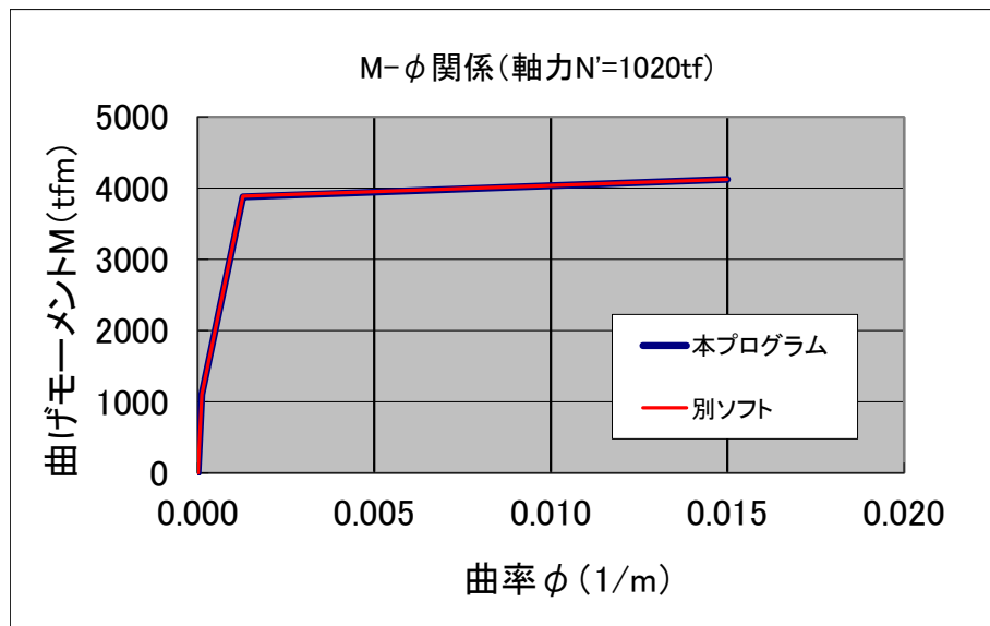
図 17-3 M- \phi 関係の計算結果
