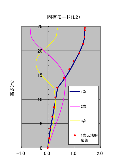
図 18-1 地盤の固有震動モードの計算例
