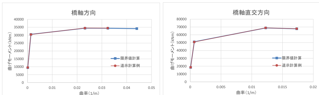
図 20-2 道示 V に基づく M-\phi 限界値の計算例（矩形断面）
