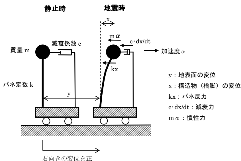
図 6-1 一自由度系振動モデル
