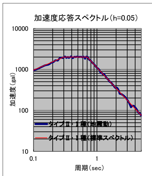
図 17-1 計算例
