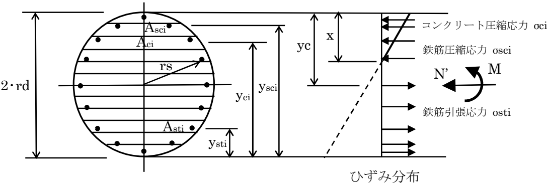
図 22-1 応力度計算の断面仮定
