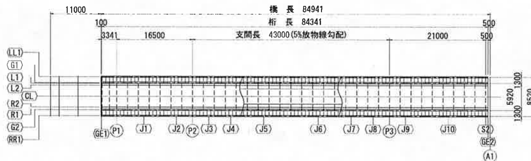
平面図
