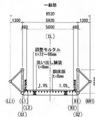
断面図
