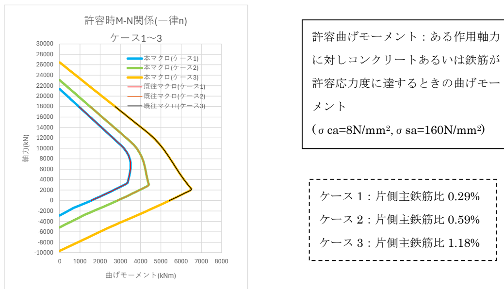
図 2-1 許容時 M-N 関係
