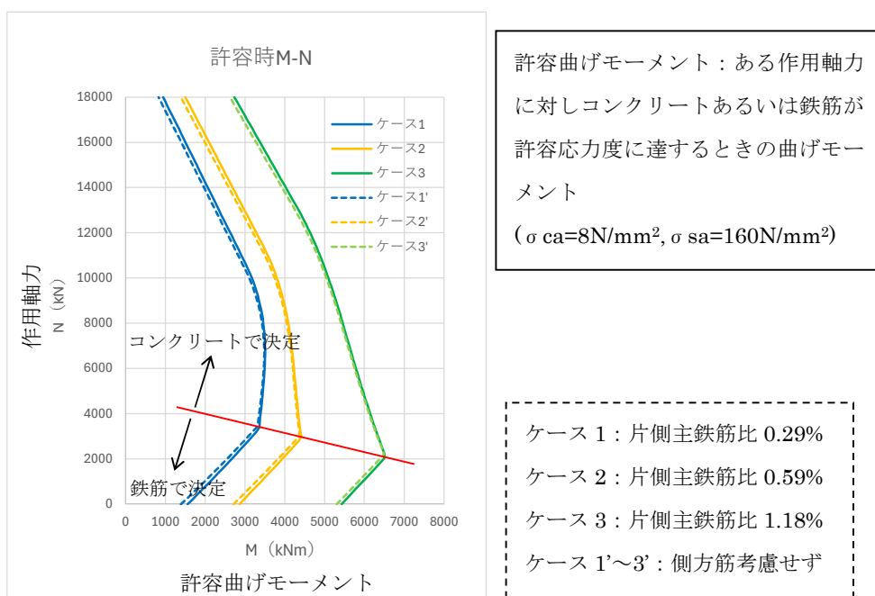
図 4-1 許容時 M-N 関係
