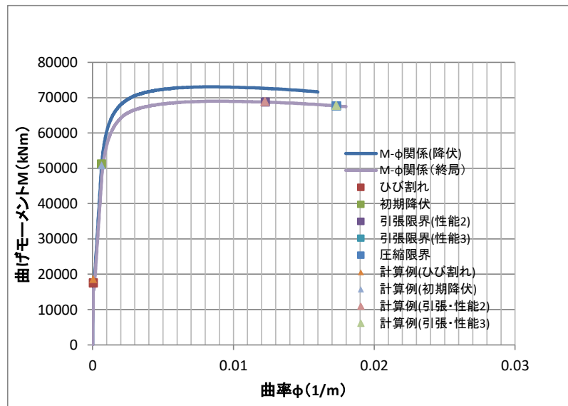
図 22-5 道示Vに基づく M - \phi 関係の計算例（矩形断面・橋軸直角方向）
