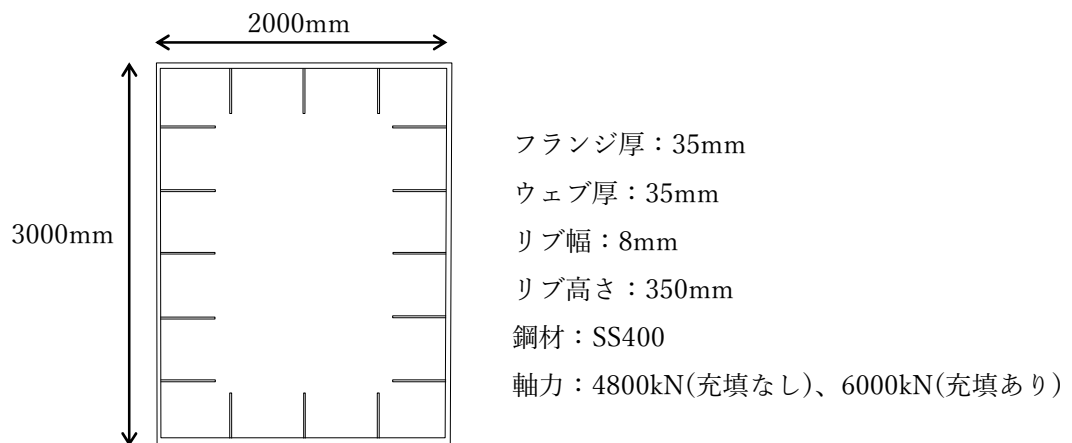
図 23-1 計算対象とした矩形鋼断面
