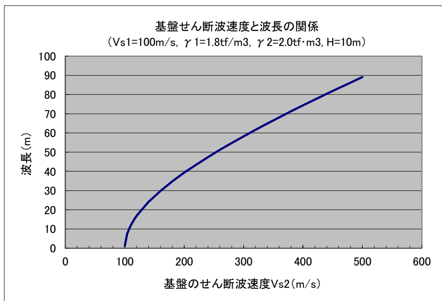
図 20-2 地盤変位波長の計算例
