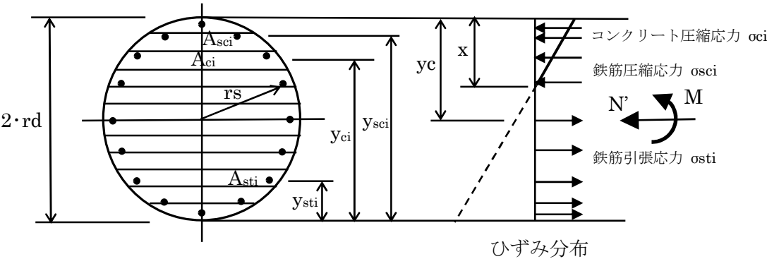
図 24-1 応力度計算の断面仮定
