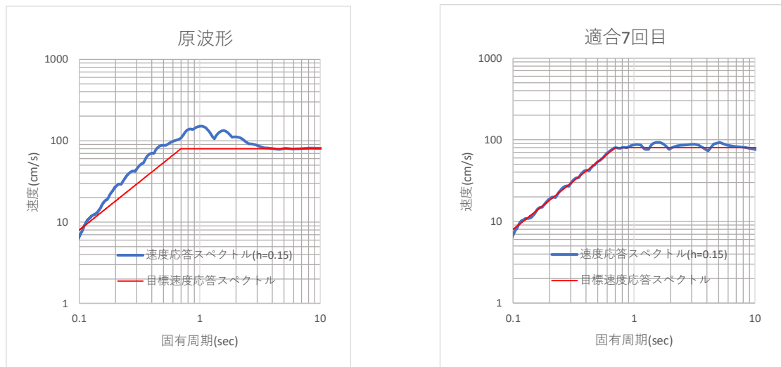
図 28-1 目標応答スペクトルとの適合
