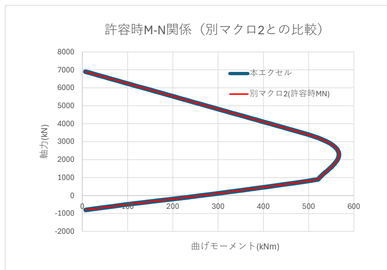
図 1-1 M-N 関係
