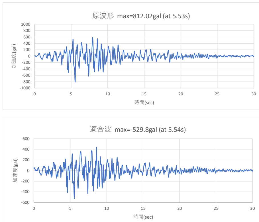
図 28-2 原波形と適合波形
