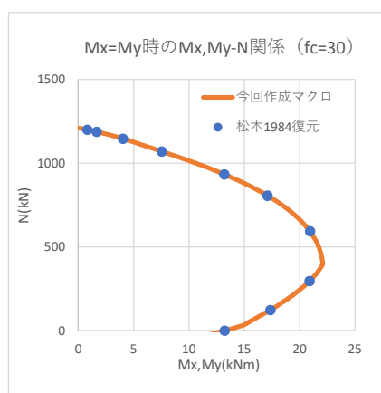
図 15-2 M_x, M_y - N 関係 ( M_x = M_y 時)
