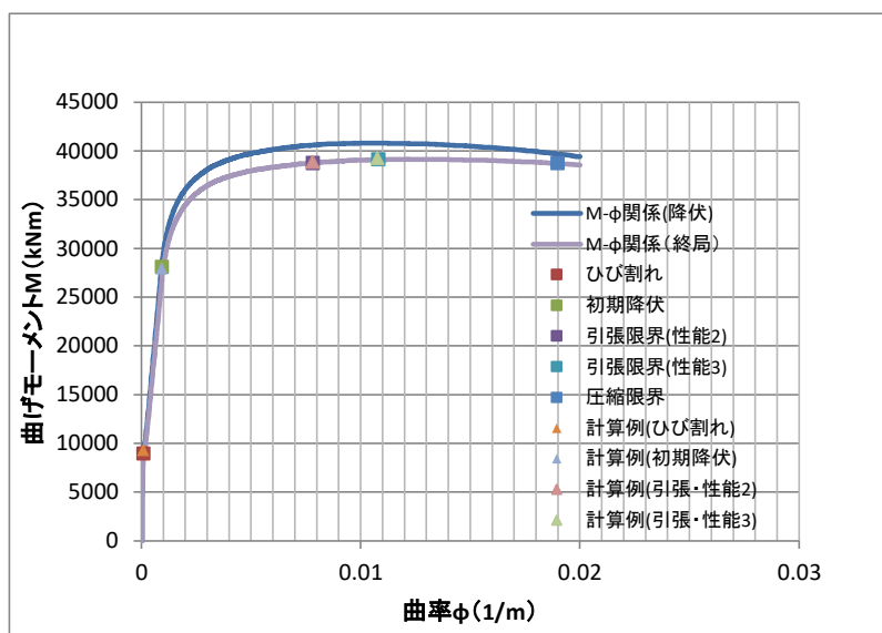
図 22-3 道示 V に基づく M-\phi 関係の計算例（円形断面）
