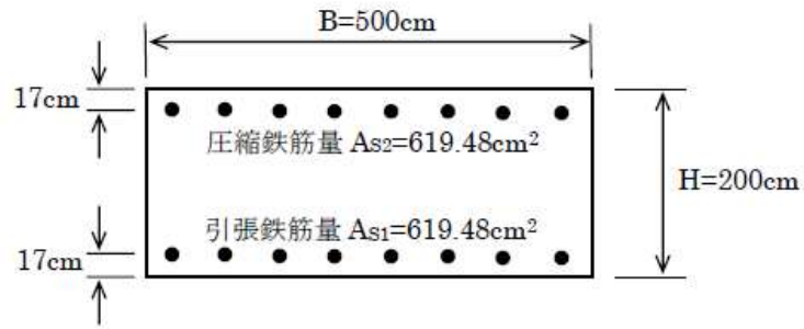
図 19-2 M- \phi 計算で仮定した RC 断面
