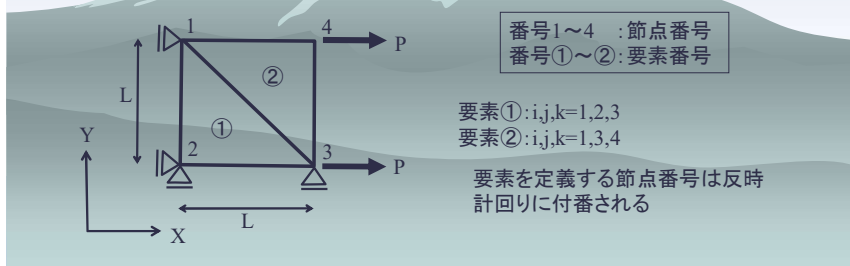
図 8-2 全体剛性マトリクスの作成
