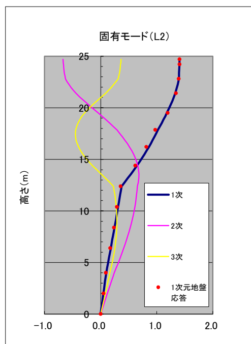
図 20-1 地盤の固有震動モードの計算例
