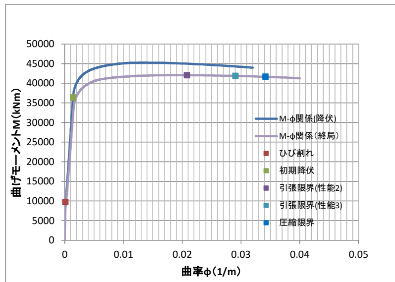
図 22-6 道示Vに基づく M - \phi 関係の計算例（小判形断面・短辺方向）
