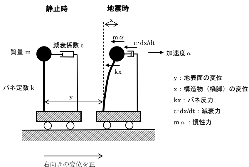
図 8-1 一自由度系振動モデル
