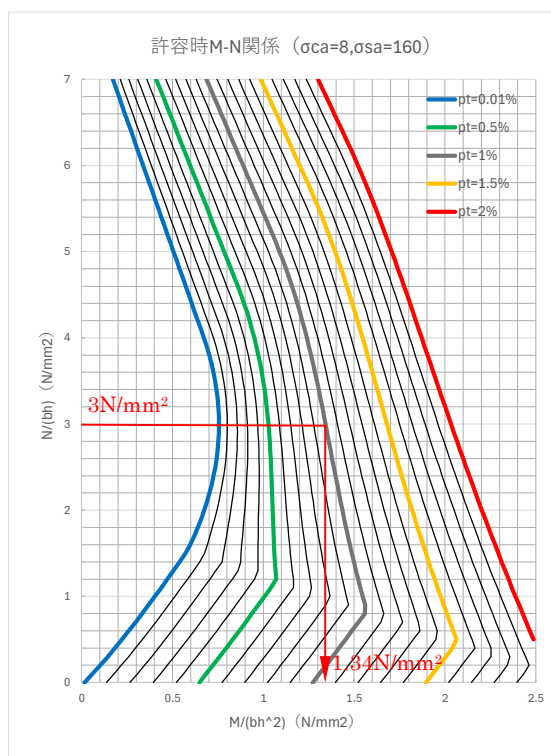
図 5-1 許容時 M-N 関係 ( \sigma_{ca}=8N/mm^2 、 \sigma_{sa}=160N/mm^2 )
