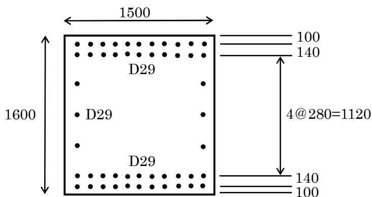
図 13-1 鉄筋配置
