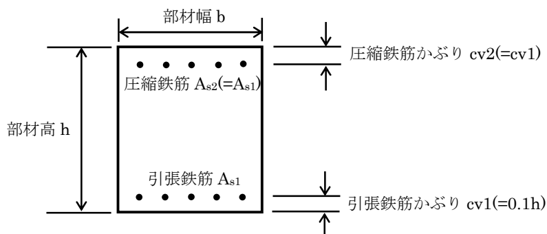
図 5-2 仮定した断面諸元
