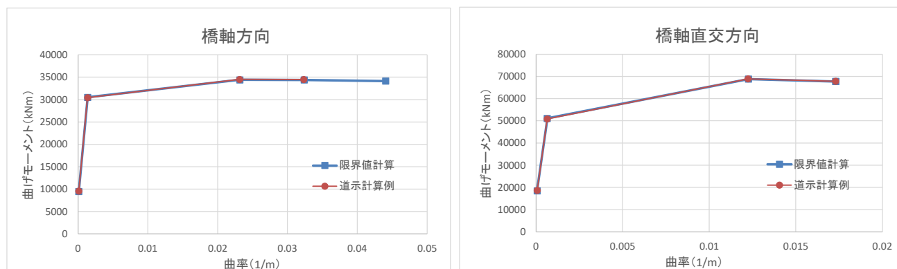
図 22-2 道示 V に基づく M-\phi 限界値の計算例（矩形断面）
