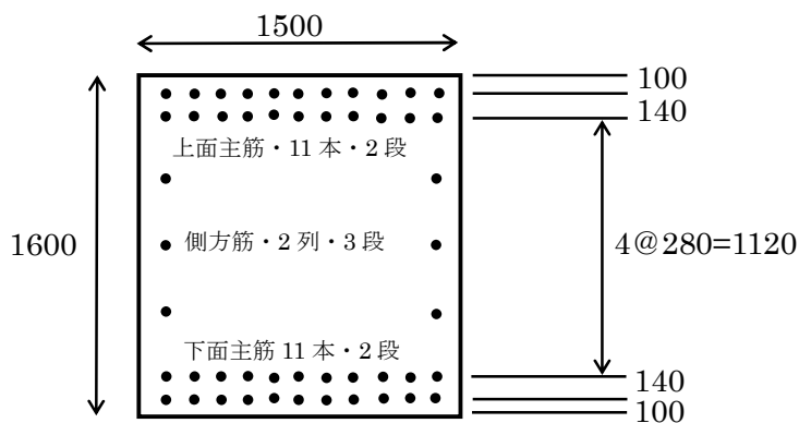
図 2-2 鉄筋配置
