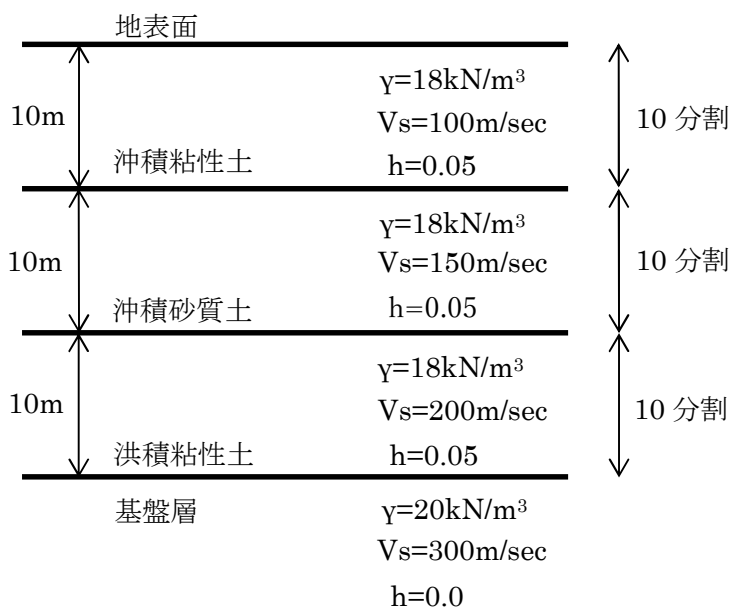
図 17-1 計算例の地層構成
