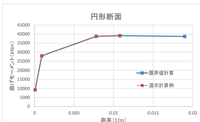
図 22-1 道示 V に基づく M-\phi 限界値の計算例（円形断面）
